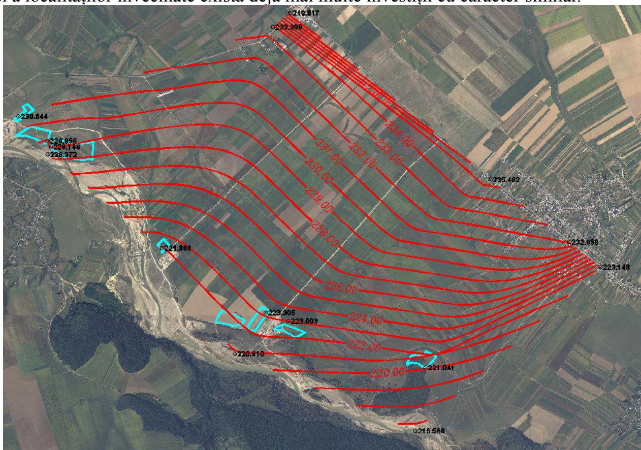
Figura 1 - Harta suprafeței piezometrice a acviferului freatic
