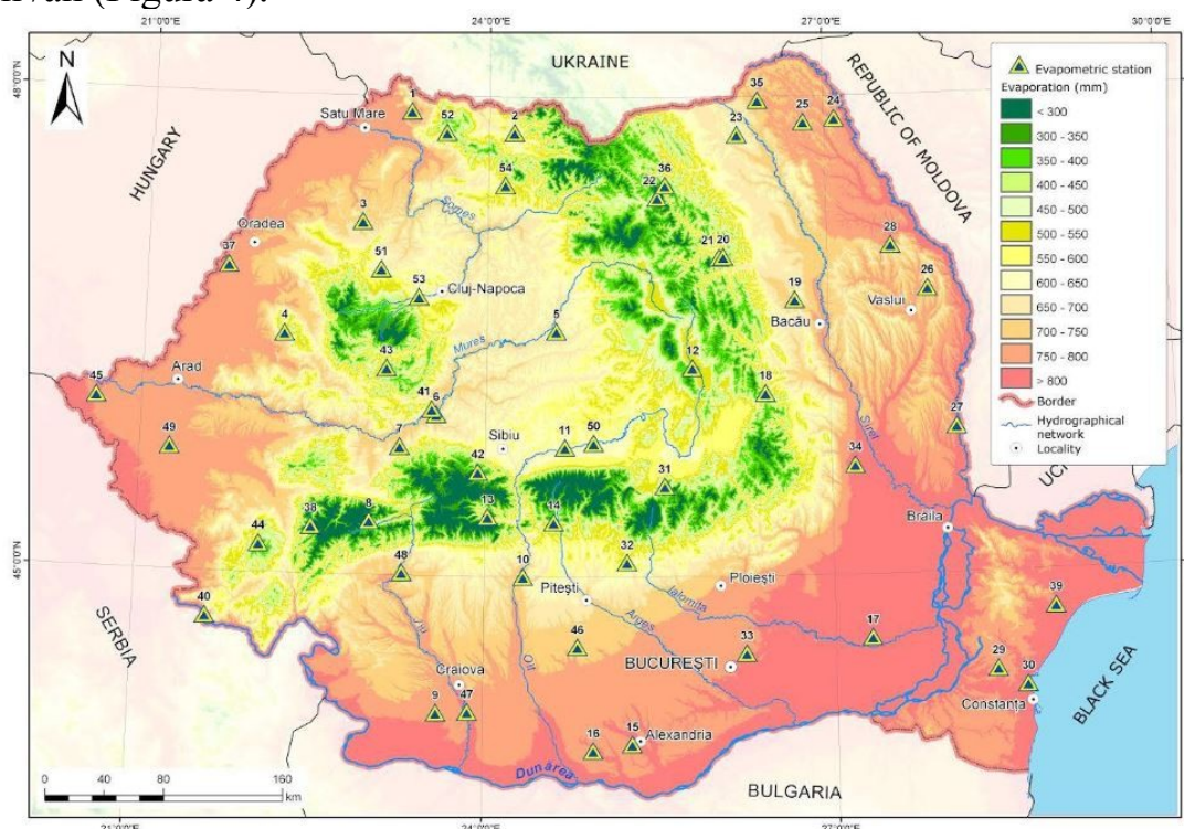
Figura 4 – Harta cu distribuția evaporăției în România
