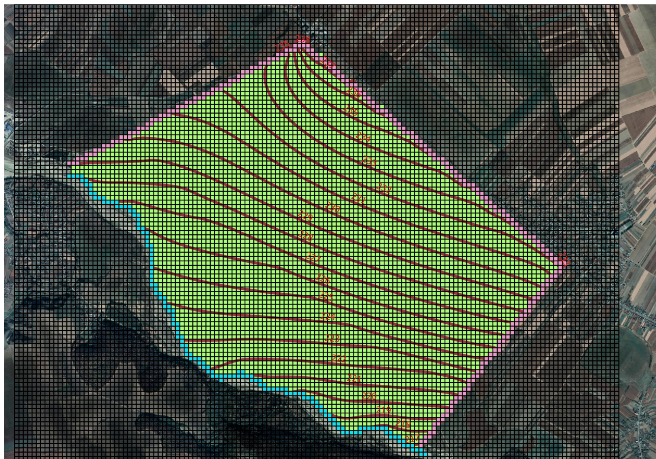
Figura 3 – Harta suprafeței piezometrice rezultată în urma procesului de calibrare
