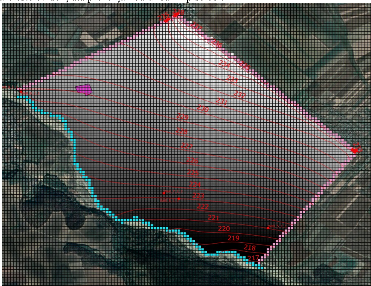
Figura 5 – Harta suprafeței piezometrice estimate
